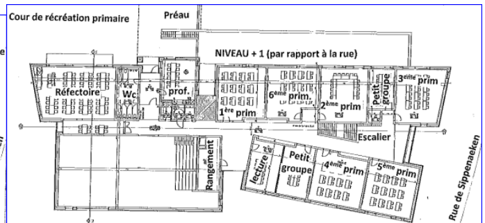
Plan du bâtiment au niveau +1 par rapport à la rue.
